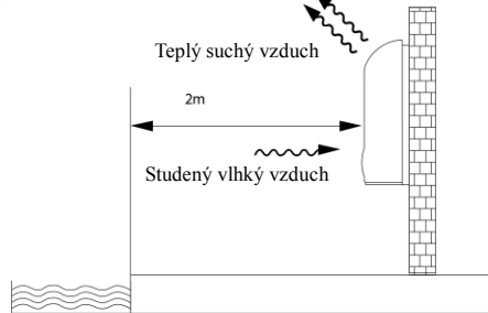
Upravovaný vzduch – instalace na zdi
